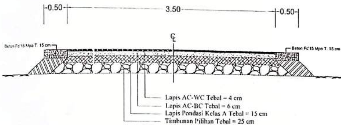
TYPICAL POTONGAN MELLINTANG JALAN STA 0+008 - 0+218 STA 0+325 - 0+350
